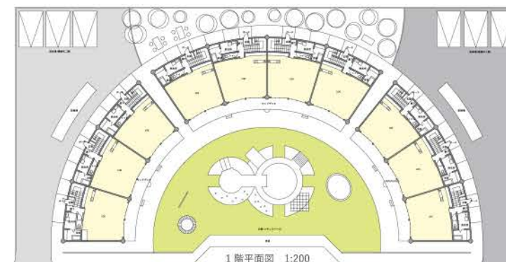
1 階平面図 1:200
