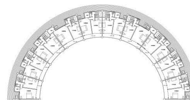
2 階平面図 1:200
